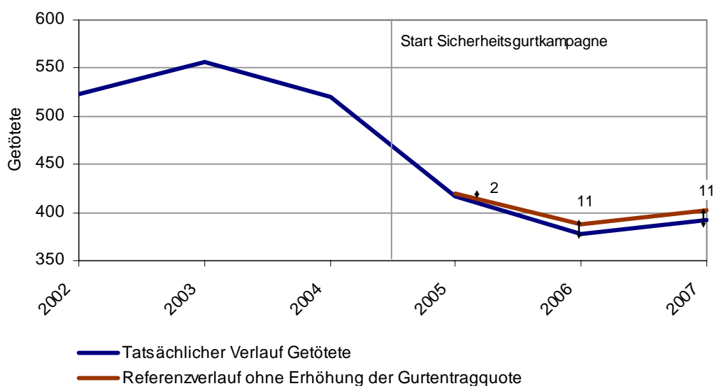
Grafik 7-6: Referenzverlauf und tatsächlicher Verlauf der Getöteten sowie vermiedene Getötete durch Erhöhung der Gurtentragquote
