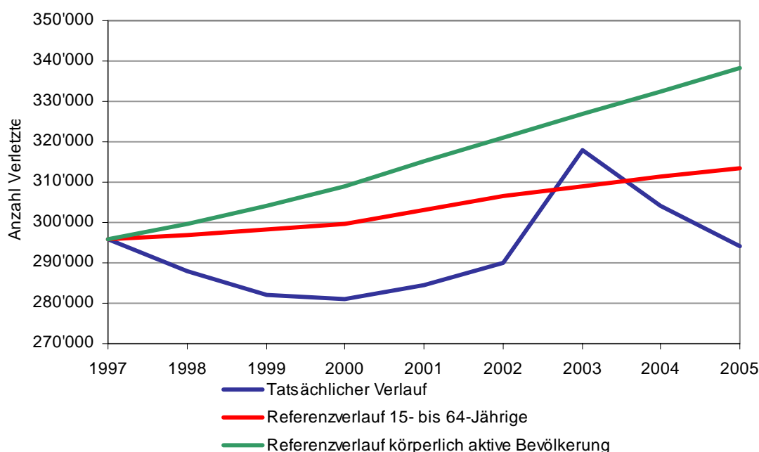
Grafik 3-10: Verletzte im NBU-Bereich Sport: Tatsächlich beobachteter Verlauf und hypothetischer Verlauf ohne Unfallverhütungsmassnahmen
