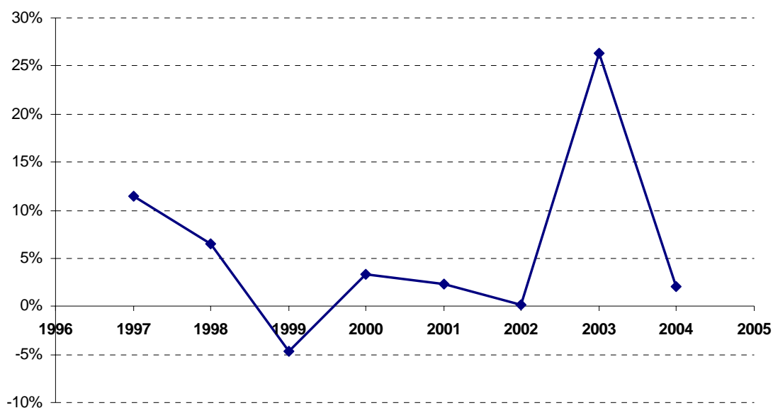
Grafik 3-11: Abweichung der jährlichen Sonnenscheindauer bezüglich dem Normwert der Jahre 1961 bis 1990
