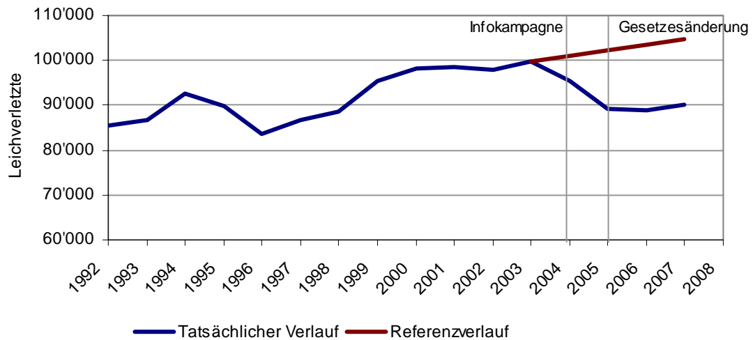
Grafik 6-4: Referenzverlauf Leichtverletzte
