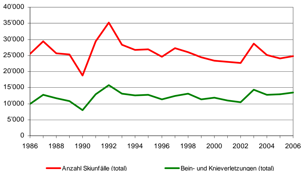
Grafik 8-1: Verletzte Skifahrer insgesamt und nach ausgewählten Verletzungsarten
