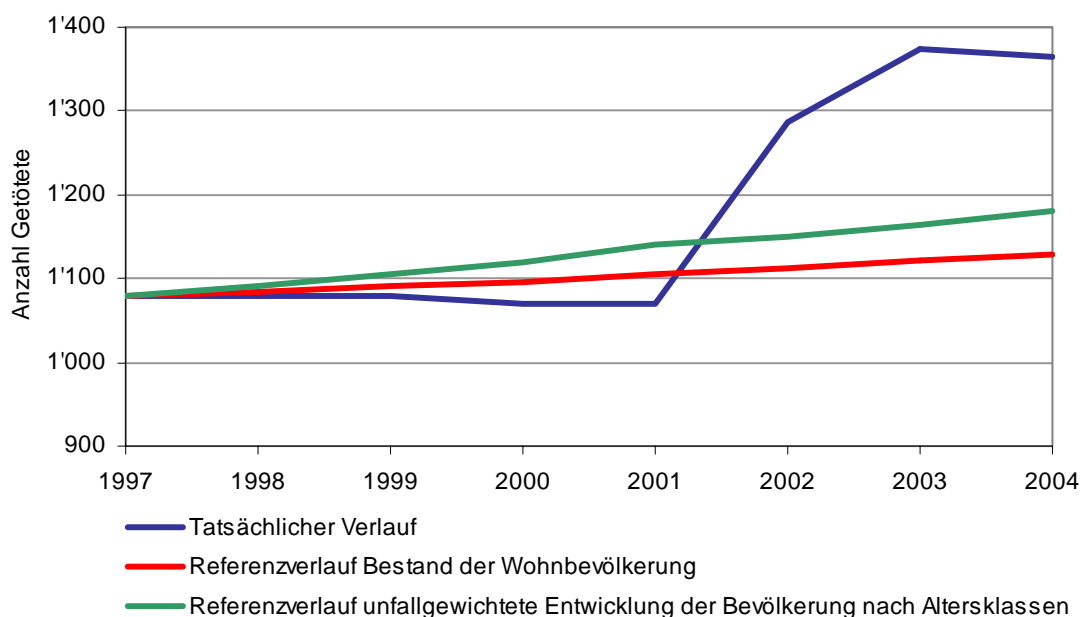
Grafik 3-13: Getötete im NBU-Bereich Haus & Freizeit: Tatsächlich beobachteter Verlauf und hypothetische Verläufe ohne Unfallverhütungsmassnahmen
