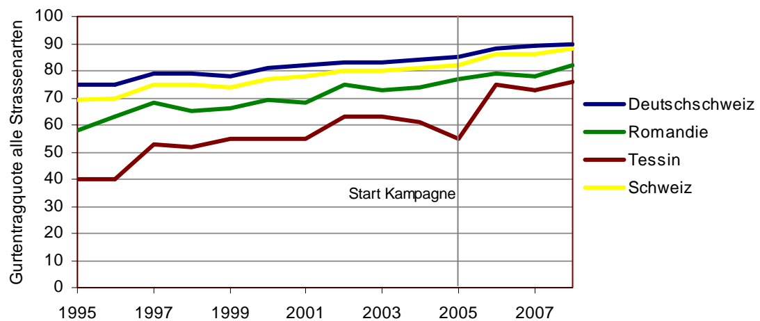
Grafik 7-1: Gurtentragquote der Personenwagenlenker, alle Strassenarten
