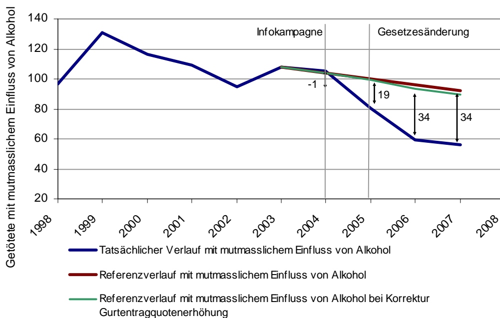
Grafik 6-9: Referenzverlauf und vermiedene Getötete bei Unfällen mit mutmasslichem Einfluss von Alkohol
