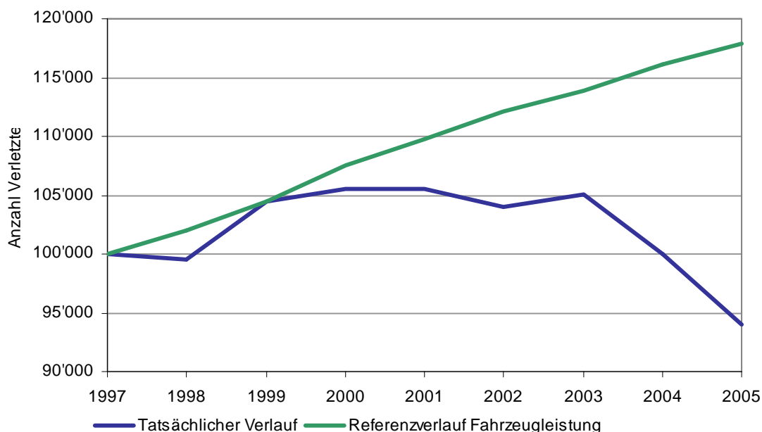
Grafik 3-8: Verletzte im NBU-Bereich Verkehr: Tatsächlich beobachteter Verlauf und hypothetischer Verlauf ohne Unfallverhütungsmassnahmen
