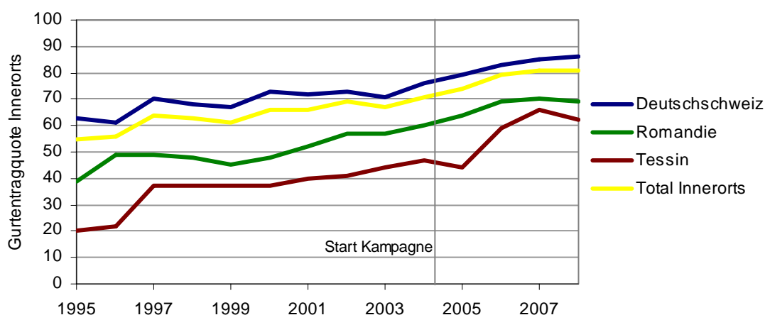
Grafik 7-4: Gurtenragquote der Personenwagenlenker, Innerorts
