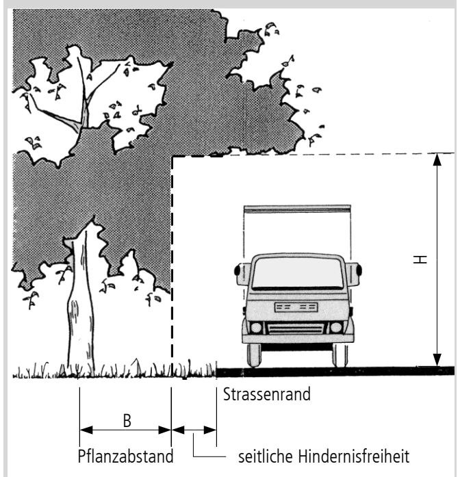
Abbildung 2 Bepflanzung entlang Strassen
