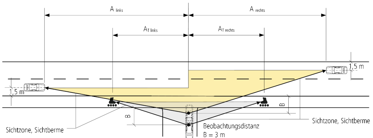
Abbildung 6 Sichtweite bei Trottoirüberfahrt
