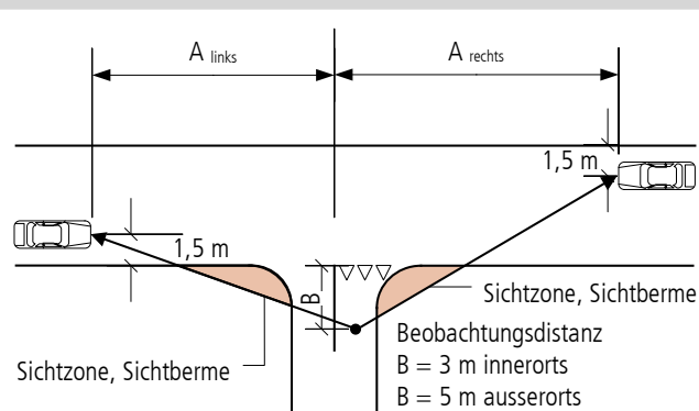
Abbildung 5 Sicht bei einer nicht vortrittsberechtigten Zufahrt
