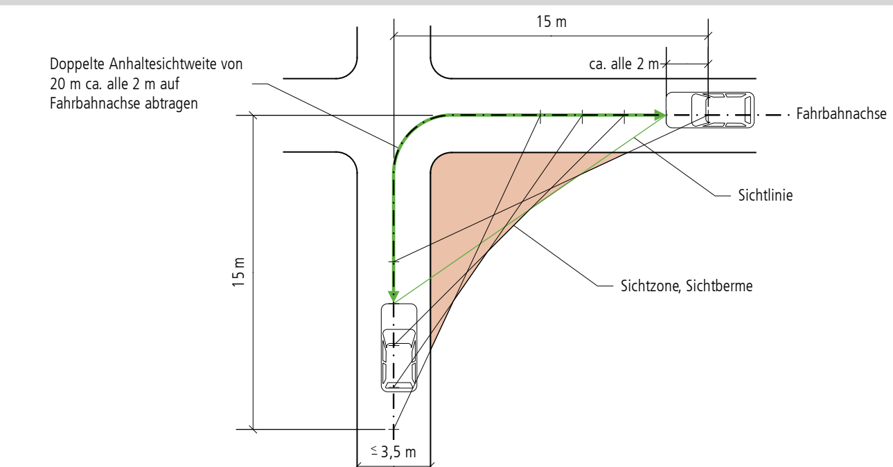
Abbildung 4 Sichtberme bei engen Verhältnissen
