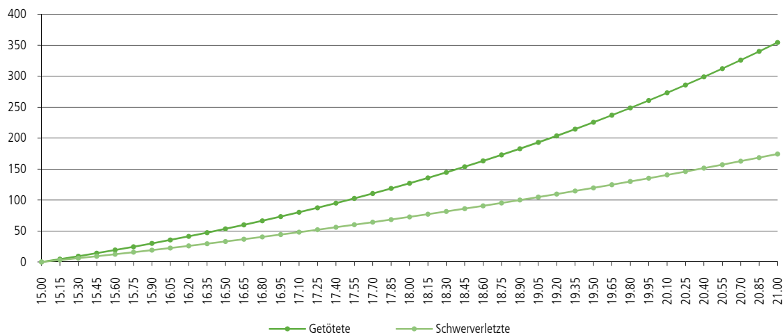
Abbildung 4 Zunahme der Anzahl Getöteten und Schwerverletzten in Abhängigkeit der Durchschnittsgeschwindigkeit (nach Rücksprache mit dem Autor von [10] auf den Fahrrad-Verkehr anwendbar)
